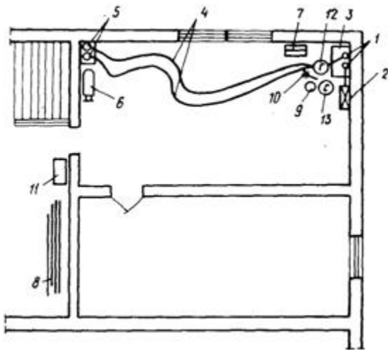
Рис. 54. Организация рабочего места
