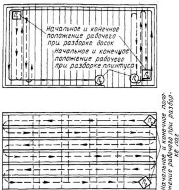
Рис. 29. Схема организации рабочего места
