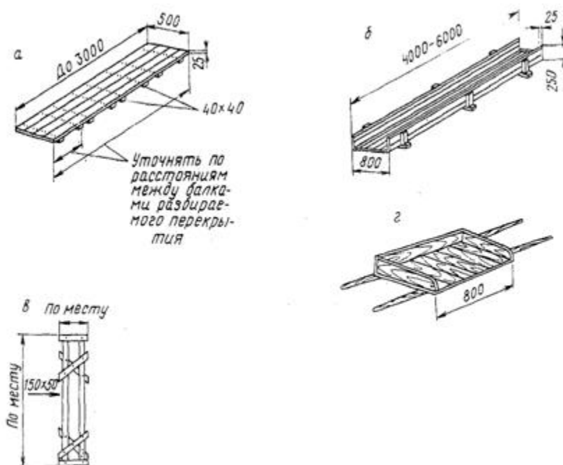
Рис. 17. Инвентарь и приспособления, применяемые при разборке деревянных перекрытий
