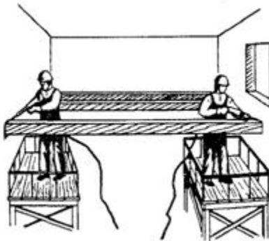
Рис. 21. Разборка подшивки
