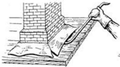
Рис. 15. Удаление открытия из кровельного железа в примыкании кровли к дымовой
