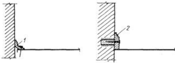
Рис. 27. Примыкание галтелей и плинтусов к стене 1 - галтель; 2 - плинтус
