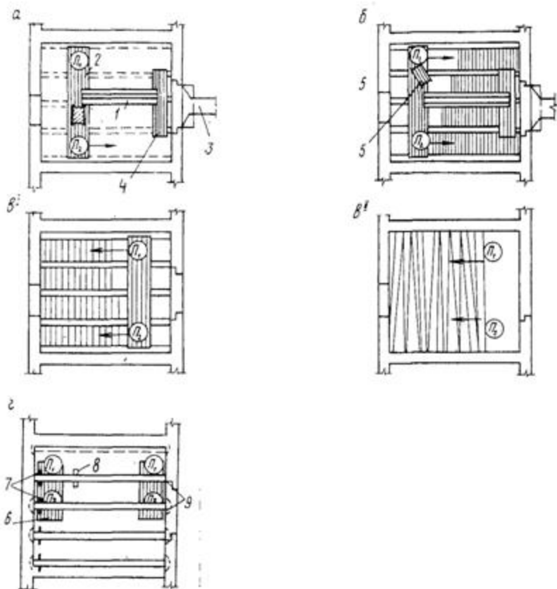
Рис. 18. Схема организации рабочего места
