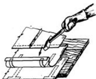
Рис. 3. Отгибание крюков и желоба
