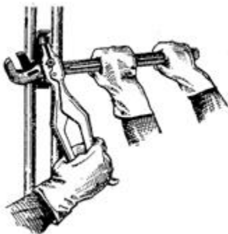
Рис. 58. Освобождение стояка от креплений
