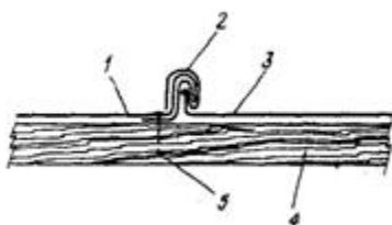
Рис. 5. Схема крепления кровельных листов кляммерами к обрешётке
