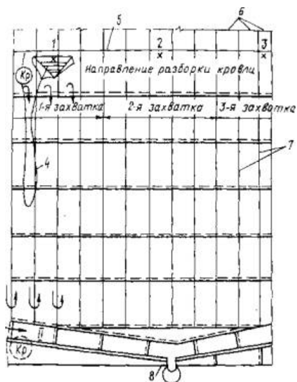
Рис. 1. Схема организации рабочего места 1, 2, 3
