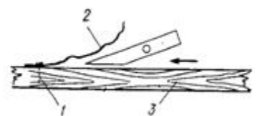
Рис. 8. Удаление кляммеры
