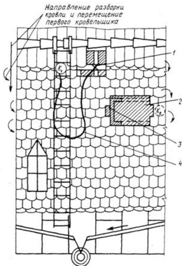
Рис. 10. схема организации рабочего места
