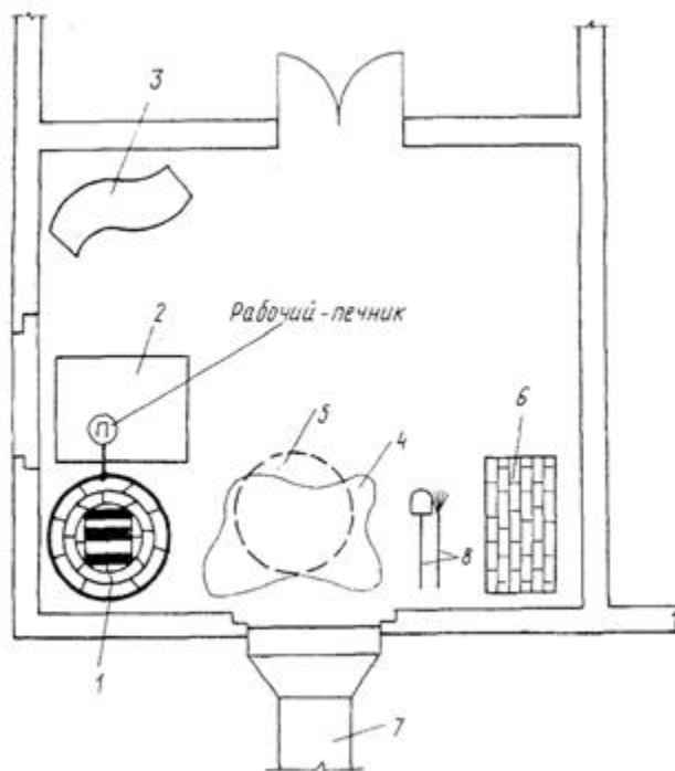
Рис. 43. Схема организации рабочего места
